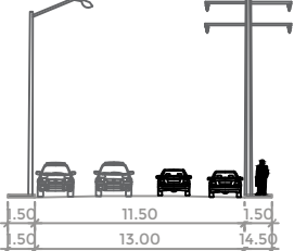
AV. PEÑA GUERRA SECCIÓN: 30.60 MTS TIPO: LOCAL
