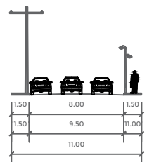
CALLE BENITO JUAREZ SECCIÓN: 11.00 MTS TIPO: LOCAL
