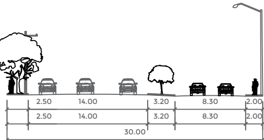
AV. BALCONES DE ANÁHUAC SECCIÓN: 30.00 MTS TIPO: SUB COLECTORA INTER BARRIOS
