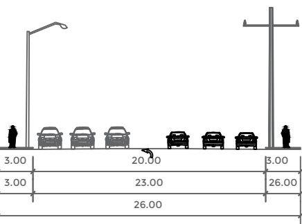
AV. DIEGO DÍAZ DE BERLANGA SECCIÓN: 26.00 MTS TRAMO: AV. DE LA JUVENTUD - AV. NOGALAR SUR TIPO: SUB COLECTORA INTERIOR
