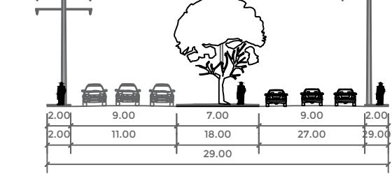
AV. CASA BLANCA SECCIÓN: 29.00 MTS TRAMO: AV. LICENCIADO ADOLFO LOPEZ MATEOS - AV. LAS TORRES TIPO: SUBCOLECTORAS INTERBARRIOS
