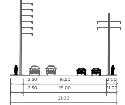
AV. FUNDIDORES SECCIÓN: 21.00 MTS TRAMO: AV. LIC. ADOLFO LOPEZ MATEOS - C. ANTIGUO CAMINO A APODACA TIPO: SUBCOLECTORAS INTERBARRIOS
