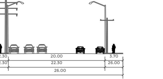
AV. PEDRO DE ALBA SECCIÓN: 20.00 MTS TIPO: SUB COLECTORA INTER BARRIOS
