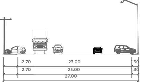
AV. ARTURO B. DE LA GARZA SECCIÓN: 27.00 MTS TIPO: SUB COLECTORA INTER BARRIOS
