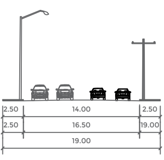
AV. SANTO DOMINGO SECCIÓN: 19.00 MTS TRAMO: MONTES BERNES - AV. DIEGO DÍAZ DE BERLANGA TIPO: SUB COLECTORA INTERIOR
