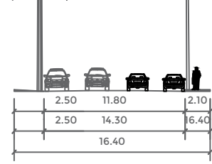
JORGE GONZÁLEZ CAMARENA SECCIÓN: 20.00 MTS TIPO: LOCAL
