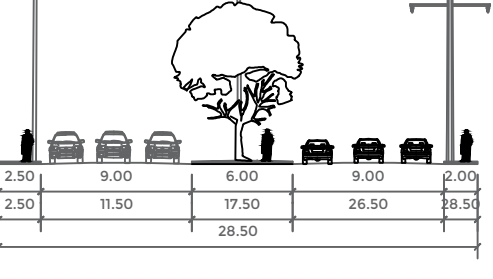
AV. CASA BLANCA SECCIÓN: 28.50 MTS TRAMO: AV. LAS TORRES - AV. MIGUEL ALEMÁN TIPO: SUBCOLECTORAS INTERBARRIOS
